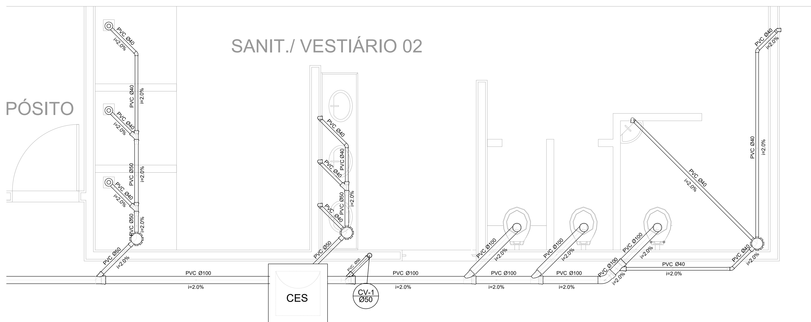
PLANTA BAIXA-PARTE 02 QUADRA PITOMBEIRA Escala: 1/25
