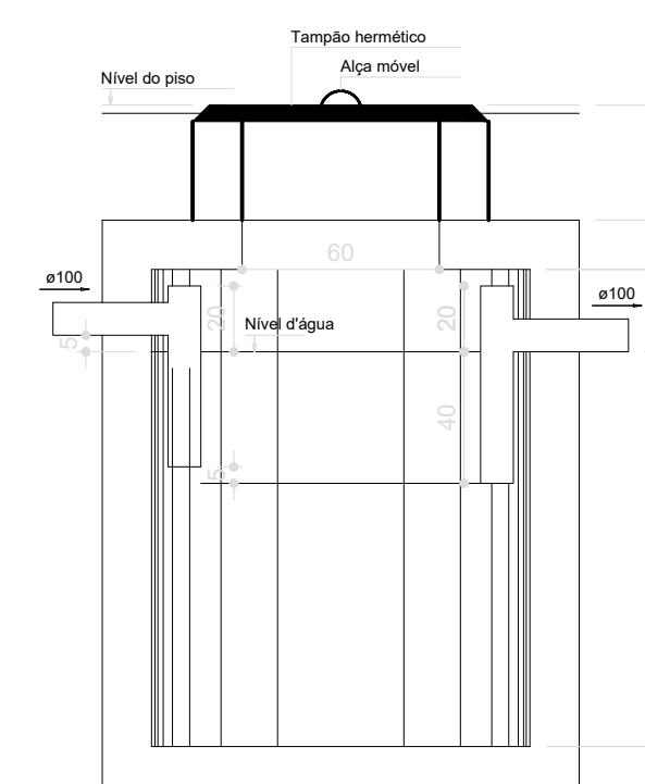
CORTE TANQUE SÉPTICO QUADRA PITOMBEIRA Escala: 1/25
