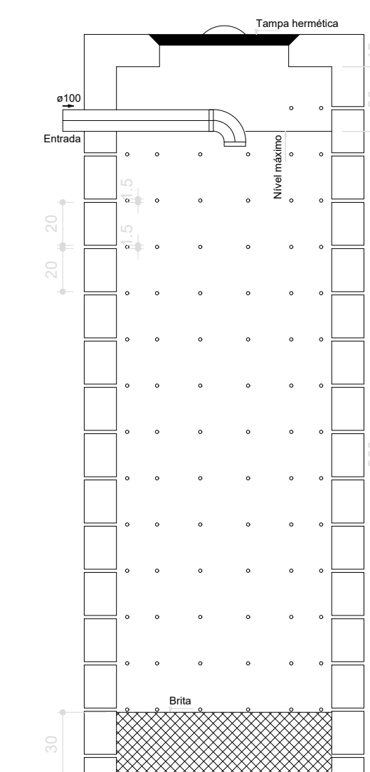
CORTE SUMIDOURO QUADRA PITOMBEIRA Escala: 1/25
