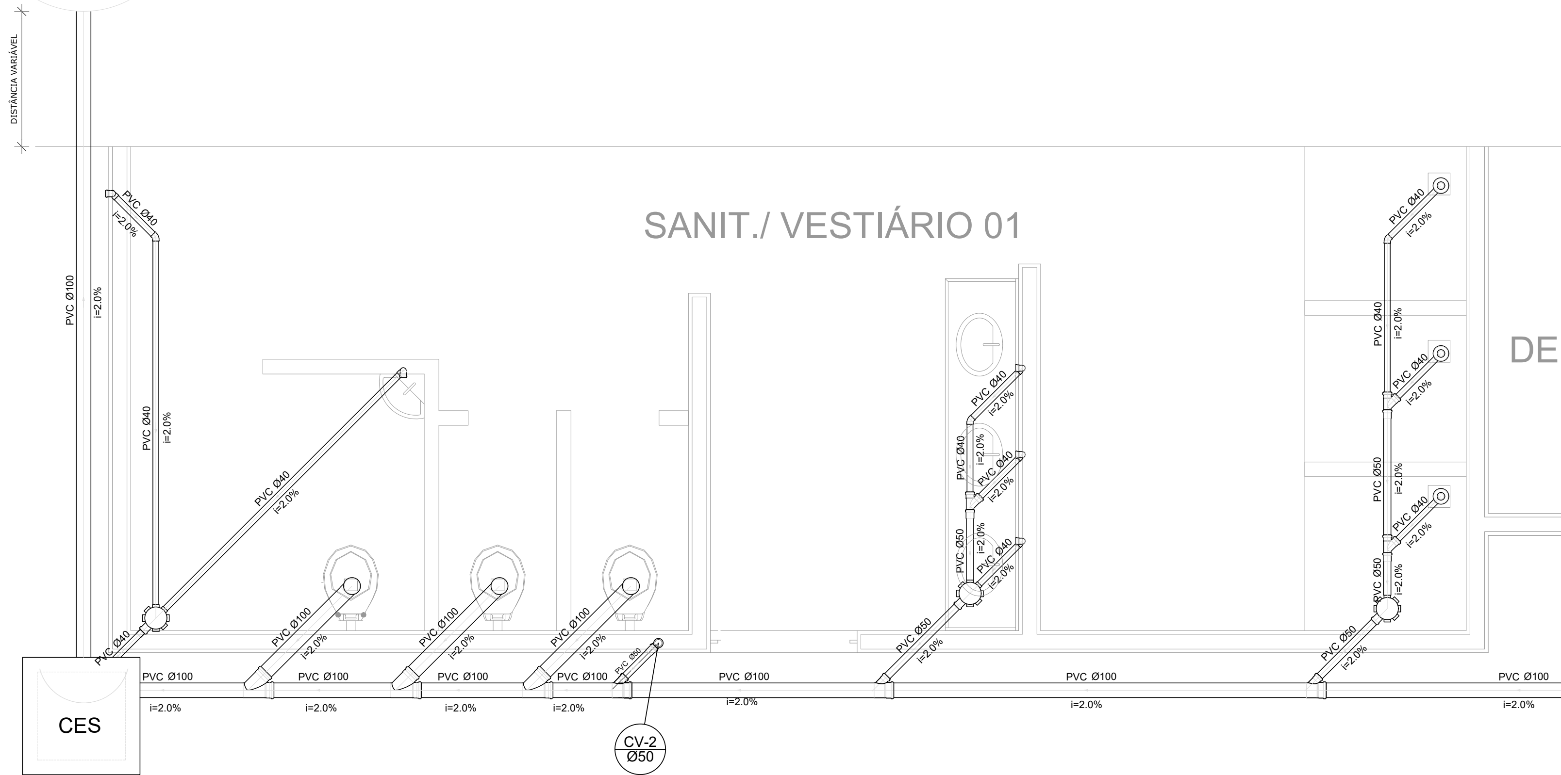
PLANTA BAIXA-PARTE 01 QUADRA PITOMBEIRA Escala: 1/25
