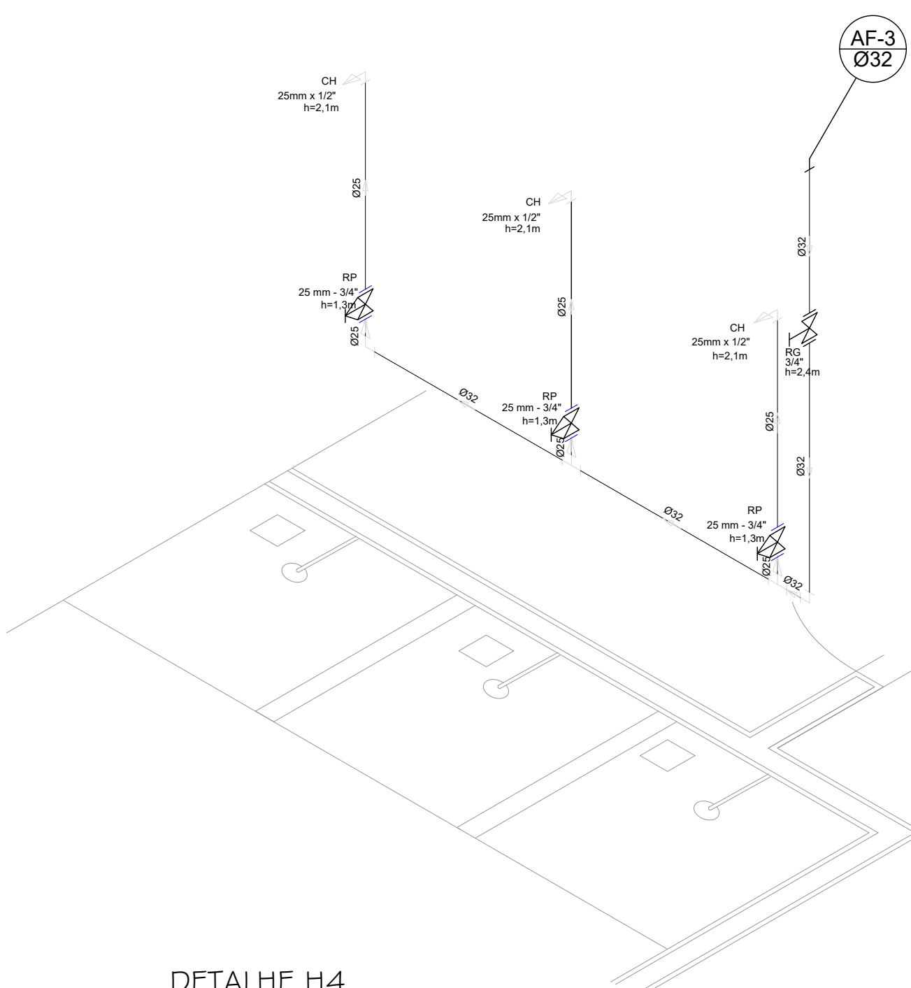
DETALHE H4 QUADRA PITOMBEIRA Escala: 1/25
