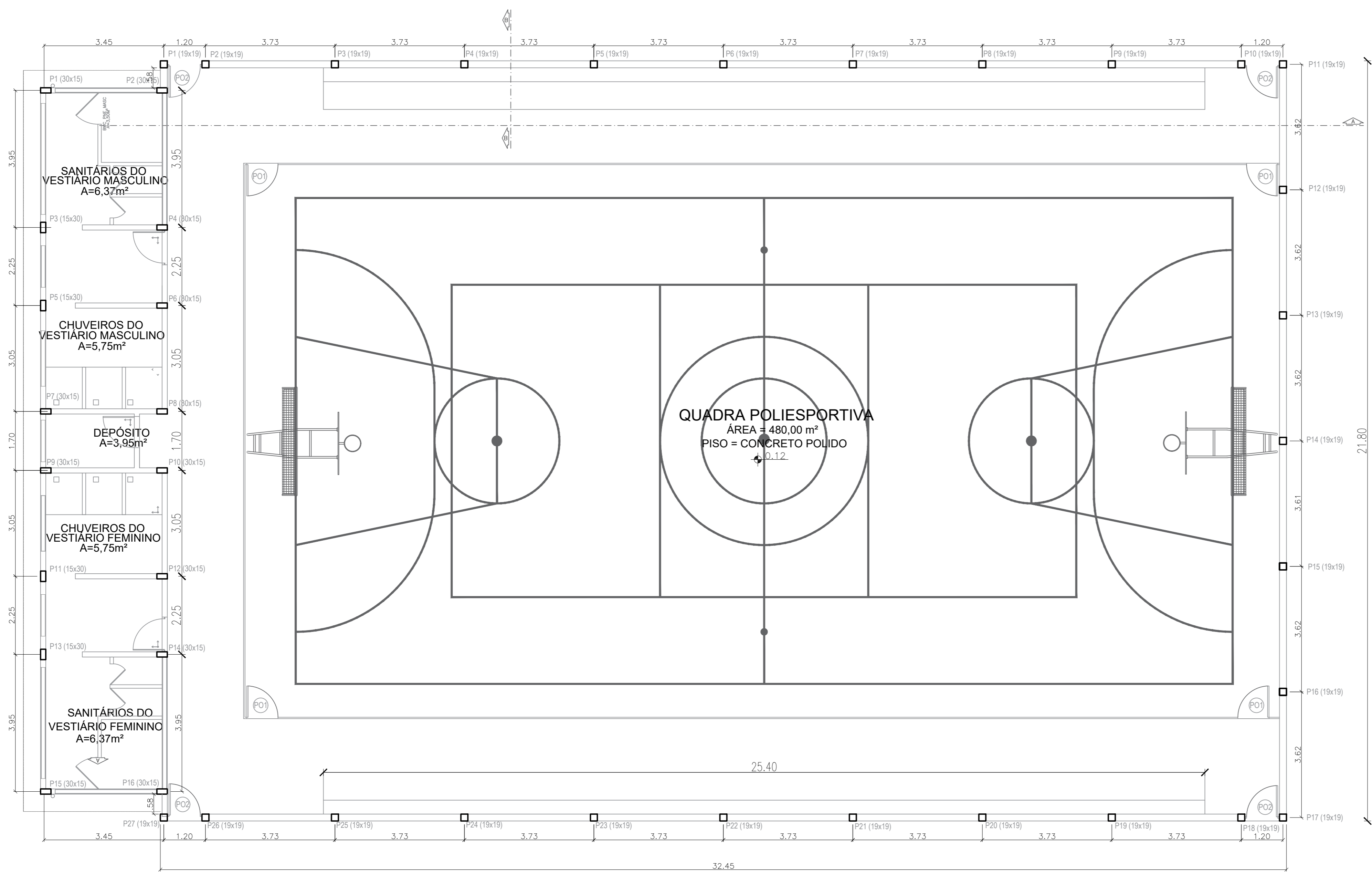
LOCAÇÃO DOS PILARES Quadra Poliesportiva - Maxaranguape / RN Escala: 1/75
