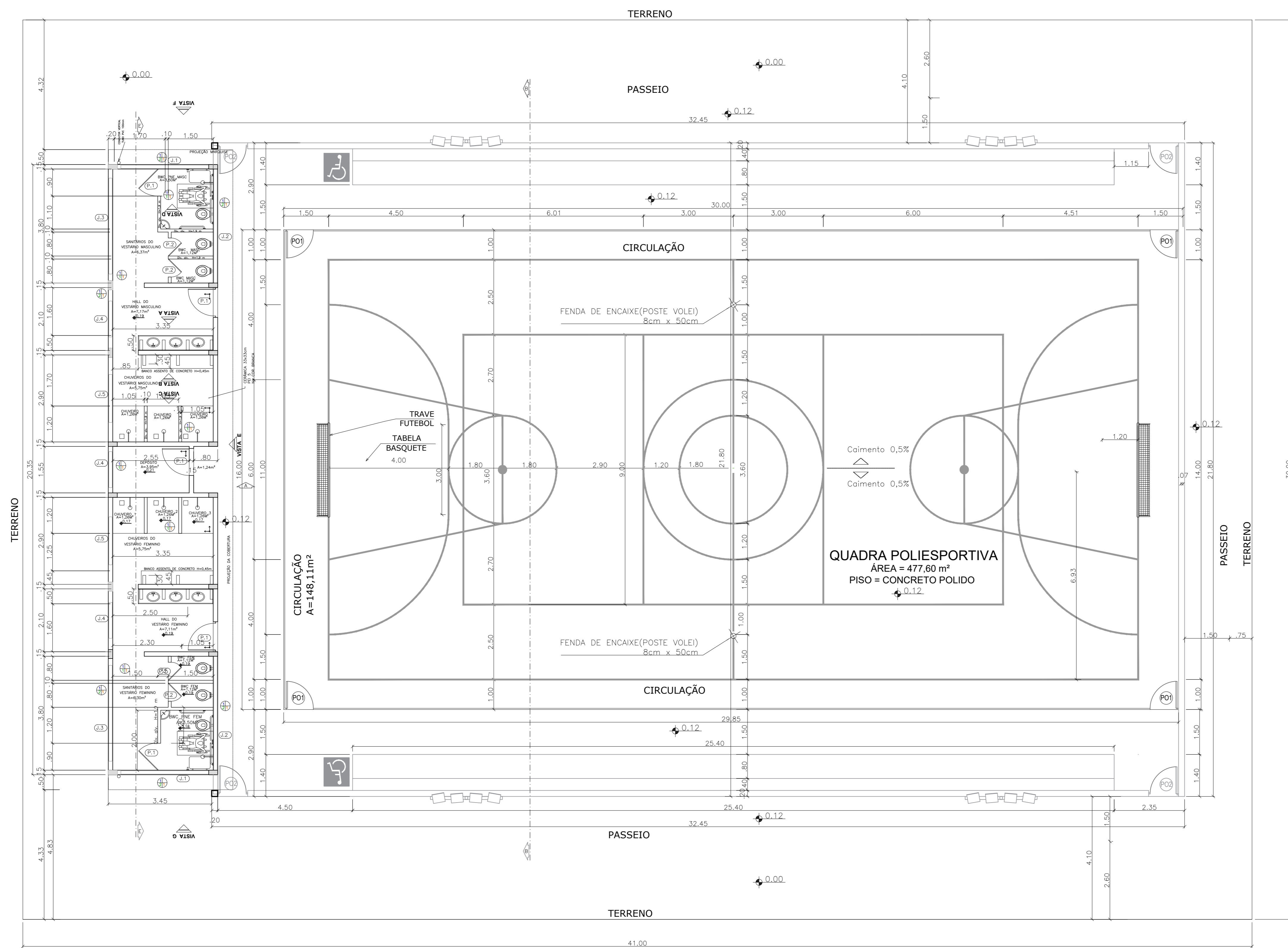
PLANTA BAIXA Quadra Poliesportiva - Maxaranguape / RN Escala: 1/75
