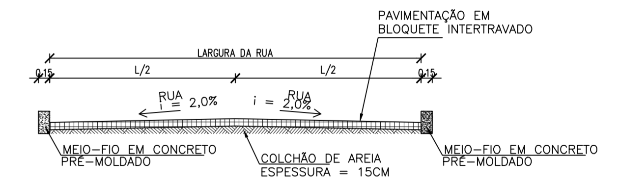
CORTE TRANSVERSAL Pavimentações, Maxaranguape/RN Escala: 1/50
