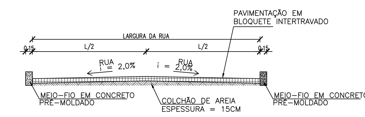
CORTE TRANSVERSAL Pavimentações, Maxaranguape/RN Escala: 1/50
