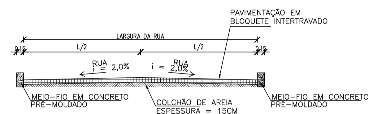
CORTE TRANSVERSAL Pavimentações, Maxaranguape/RN Escala: 1/50
